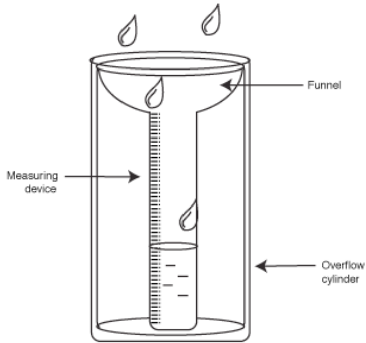
Fig. Rain Gauge
